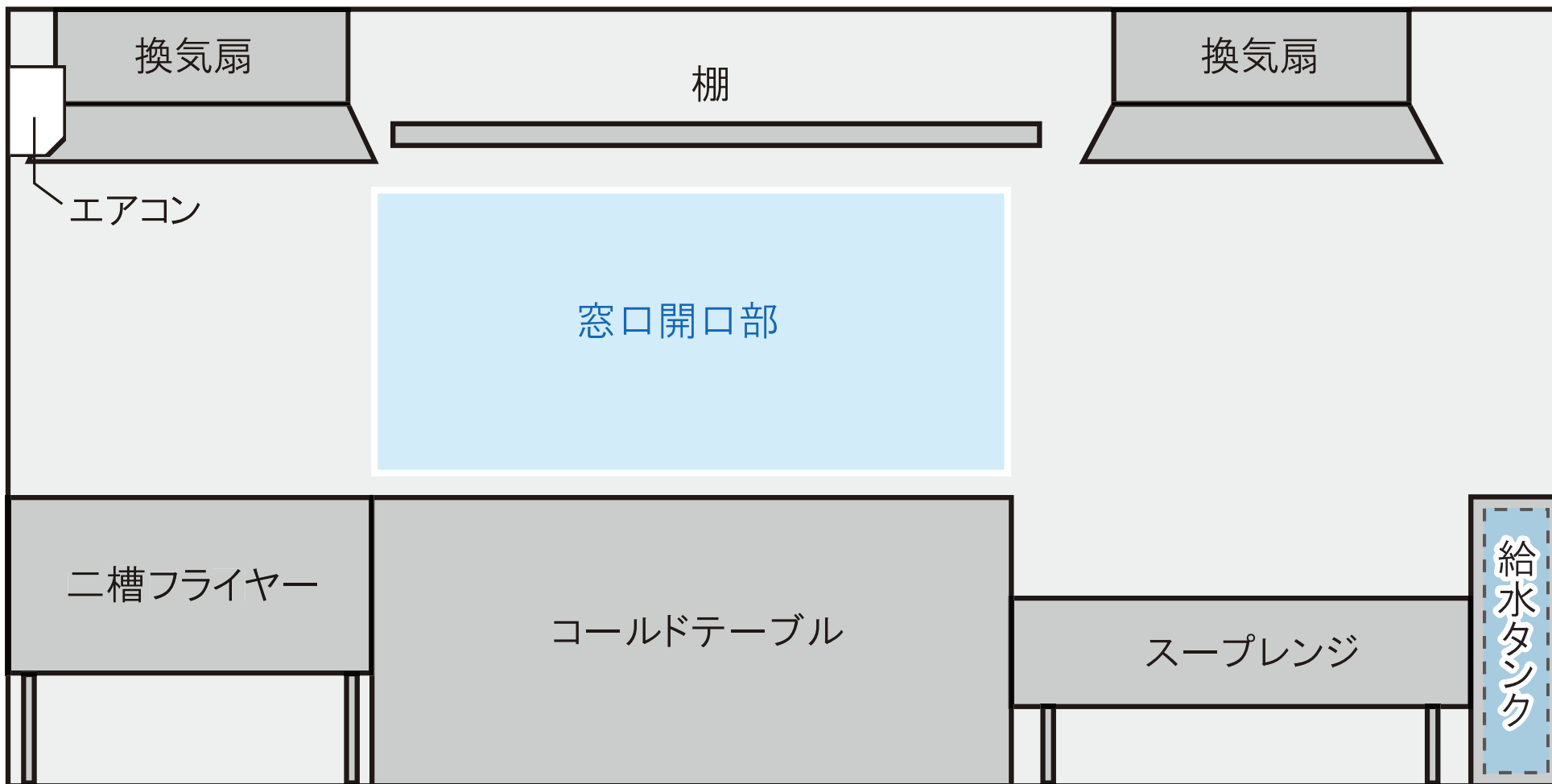
「立面図(右)」
